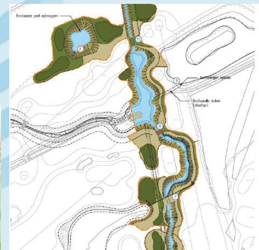
Afbeelding 4 Impressie definitief ontwerp EVZ Bleekloop
